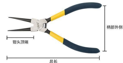
穴用直咀卡簧钳
